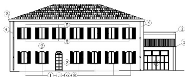
Prospetto Ovest
