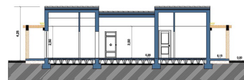
SEZIONE A-A
